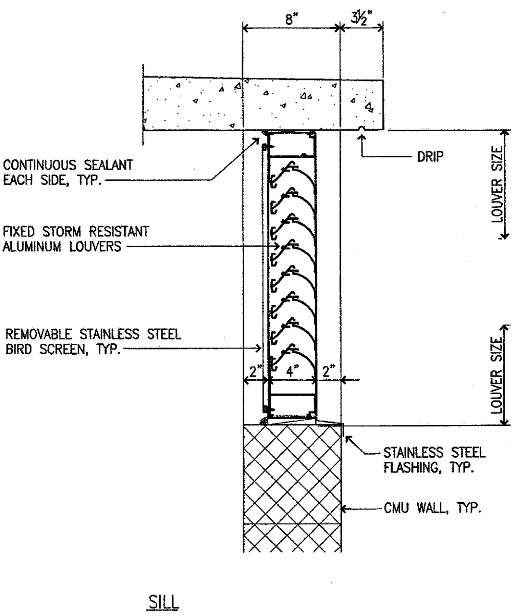
1 LOUVER SECTION AD1.1 SCALE: 1 1/2" = 1'-0"
