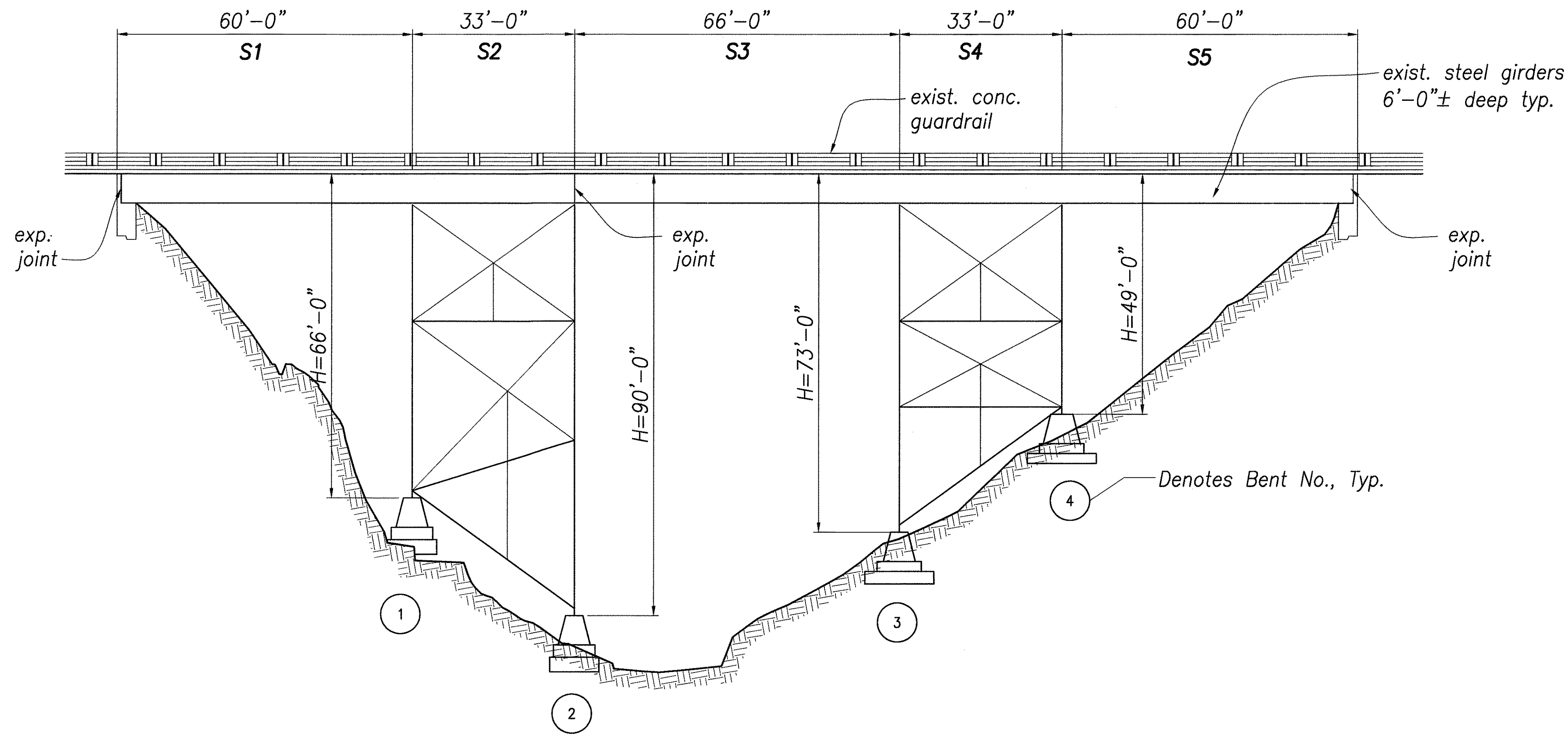
ELEVATION Scale: 1/16" = 1'-0" A 13 13
