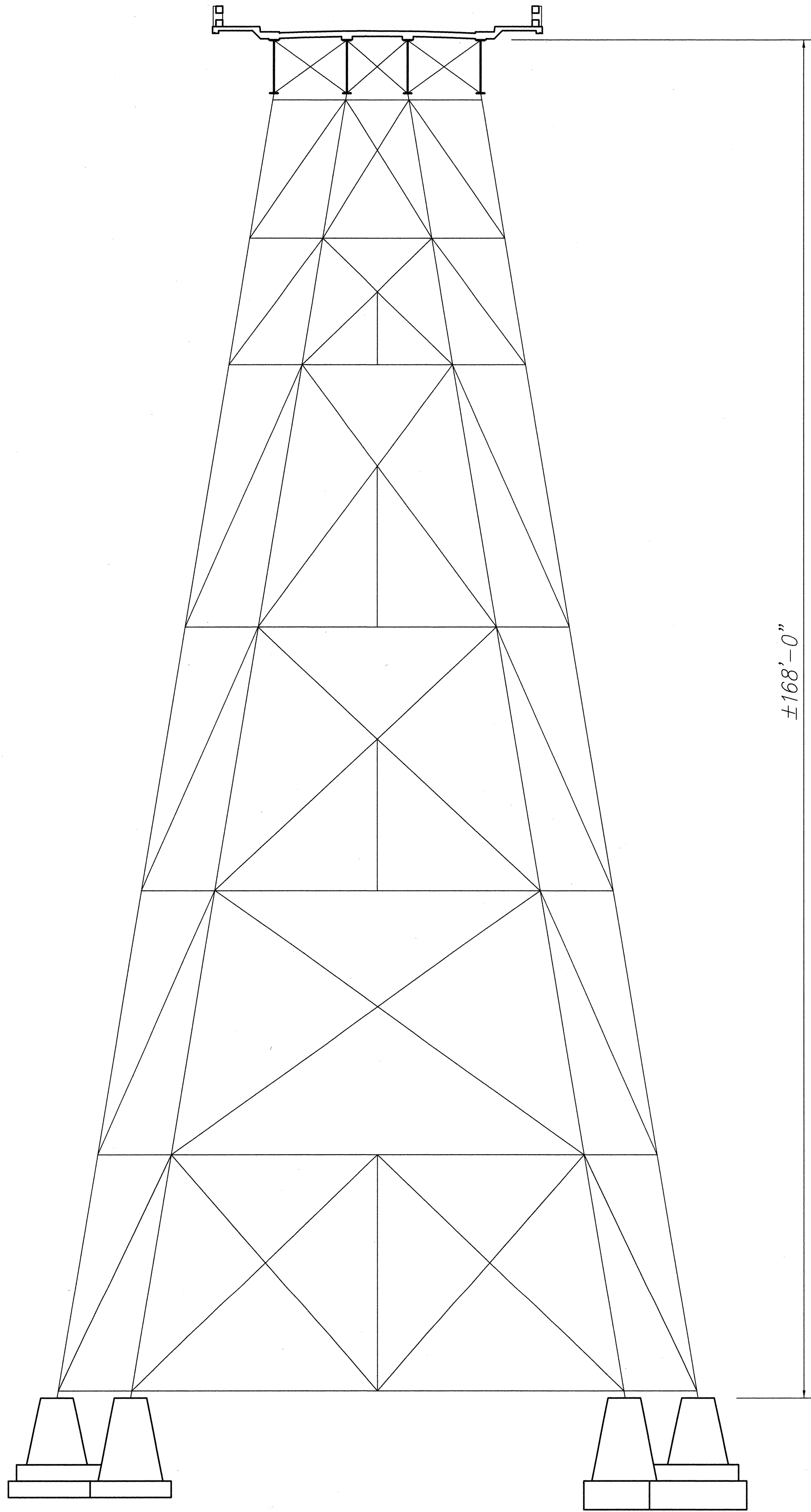
BENT #10
