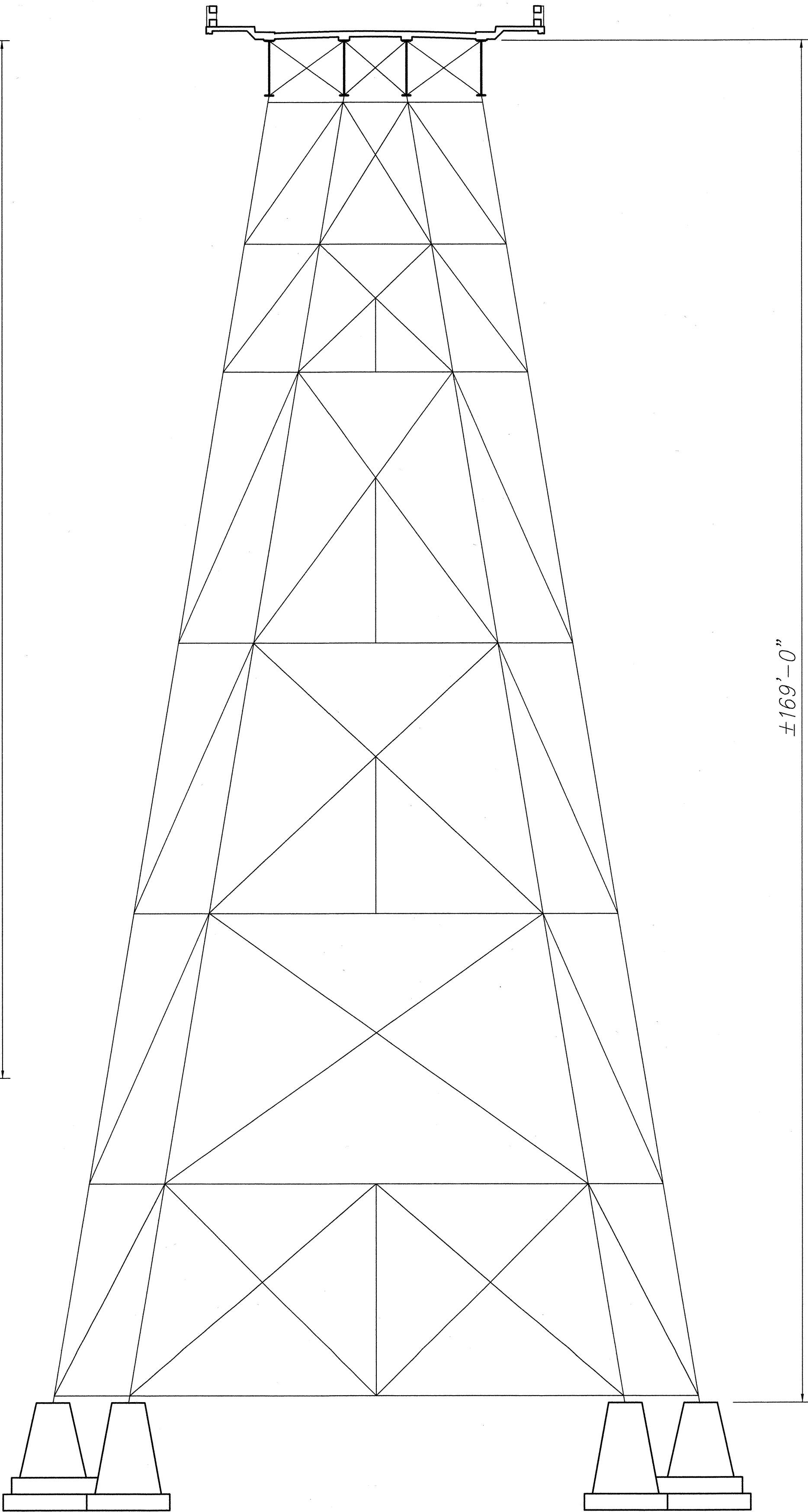
BENT #3
