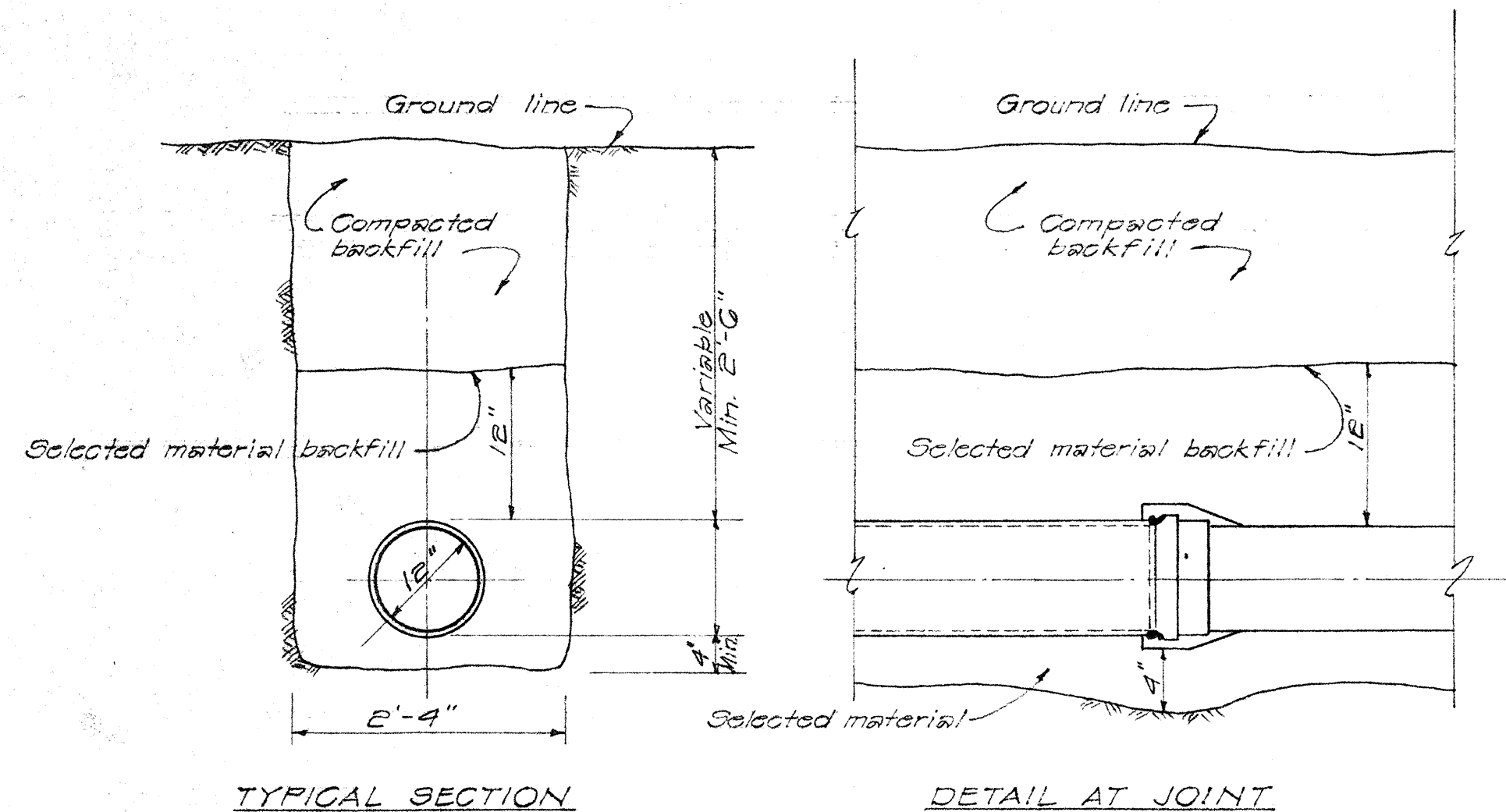
WATERLINE TRENCH DETAILS Scale: 1" = 1'-0"
