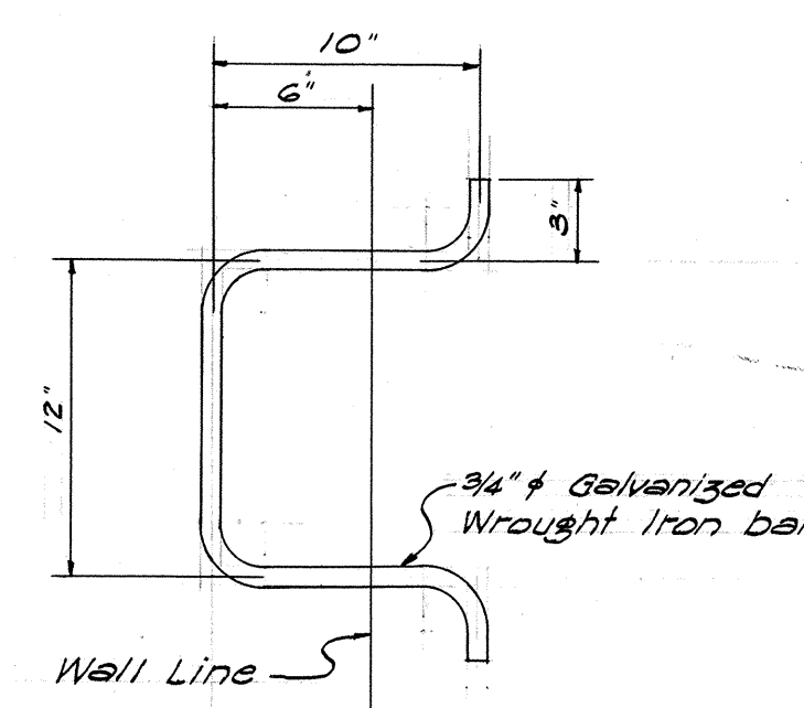
MANHOLE RUNG Scale: 1/2"=1'0"
