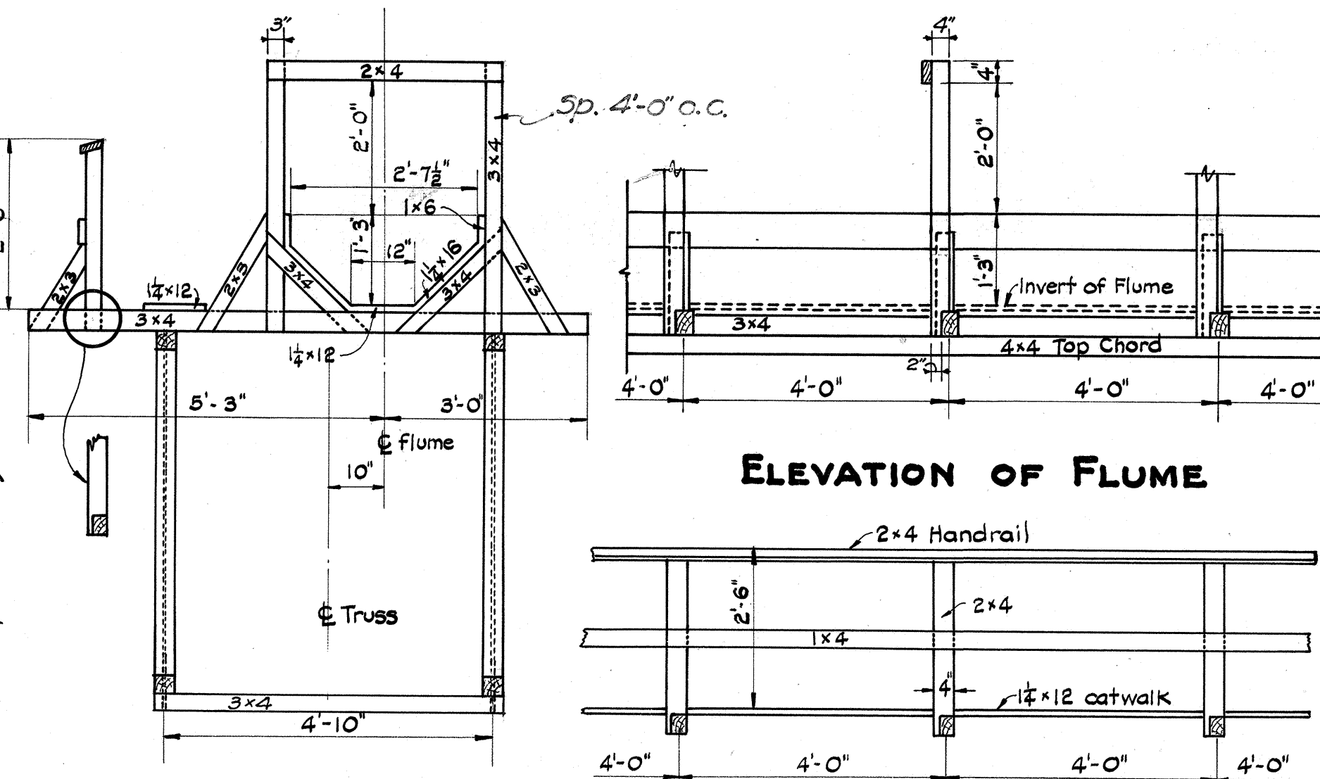
SECTION A-A Scale: \frac{1}{2}'' = 1'-0''
