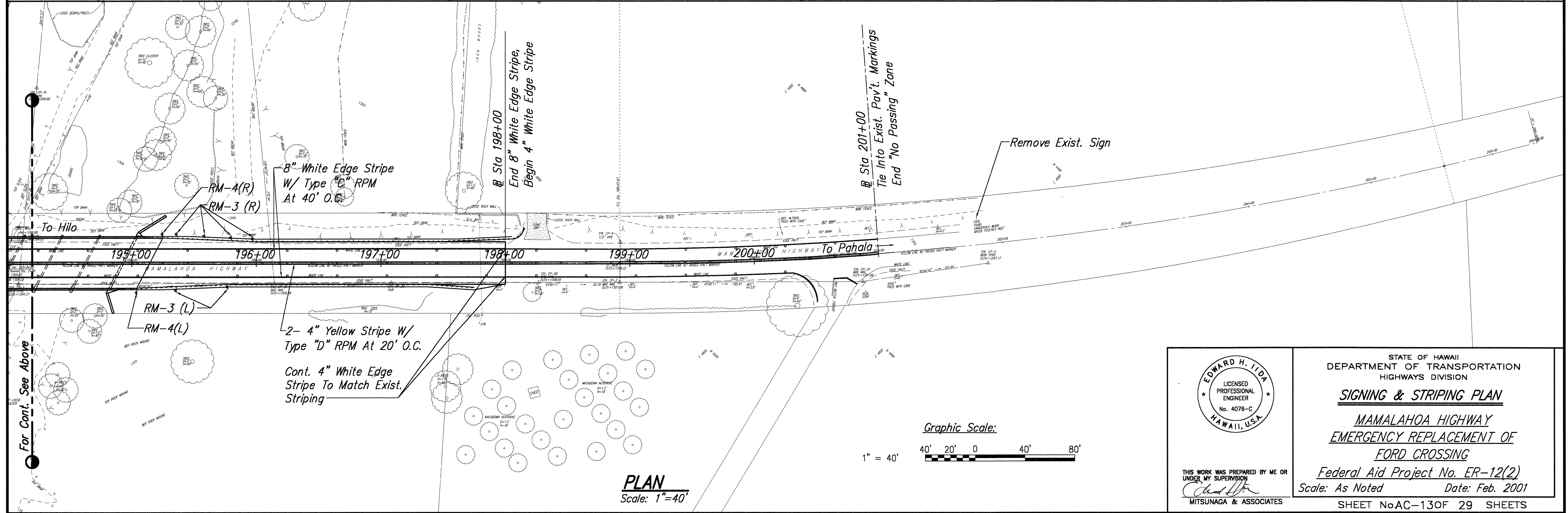
PLAN Scale: 1"=40'
