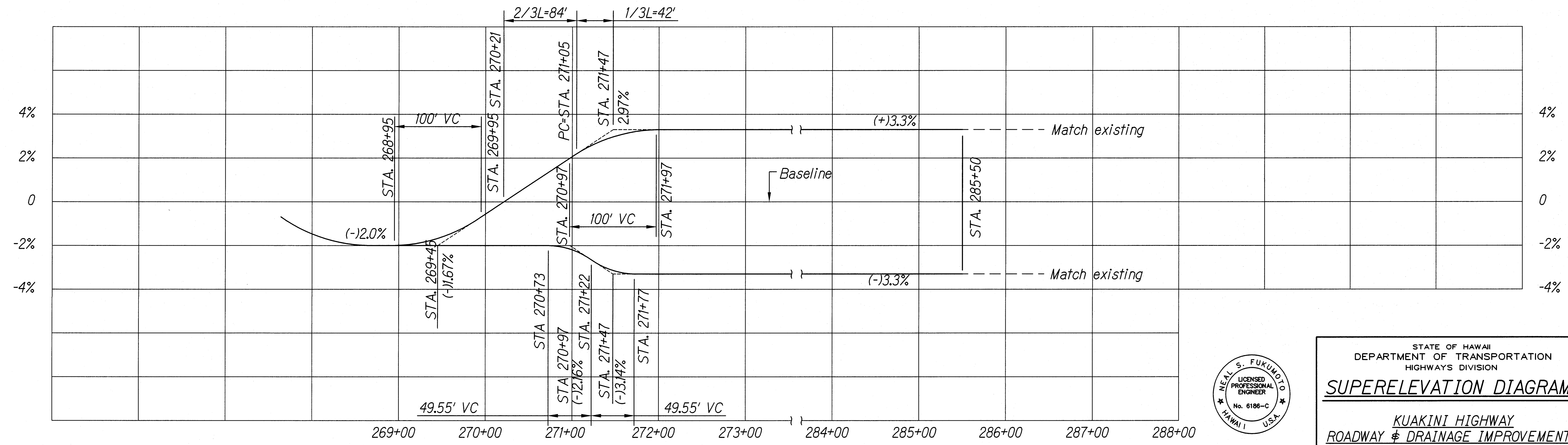
PC STA. 271+05 TO PT STA. 286+00 Scale: Horiz 1"=60' Vert 1"=2%
