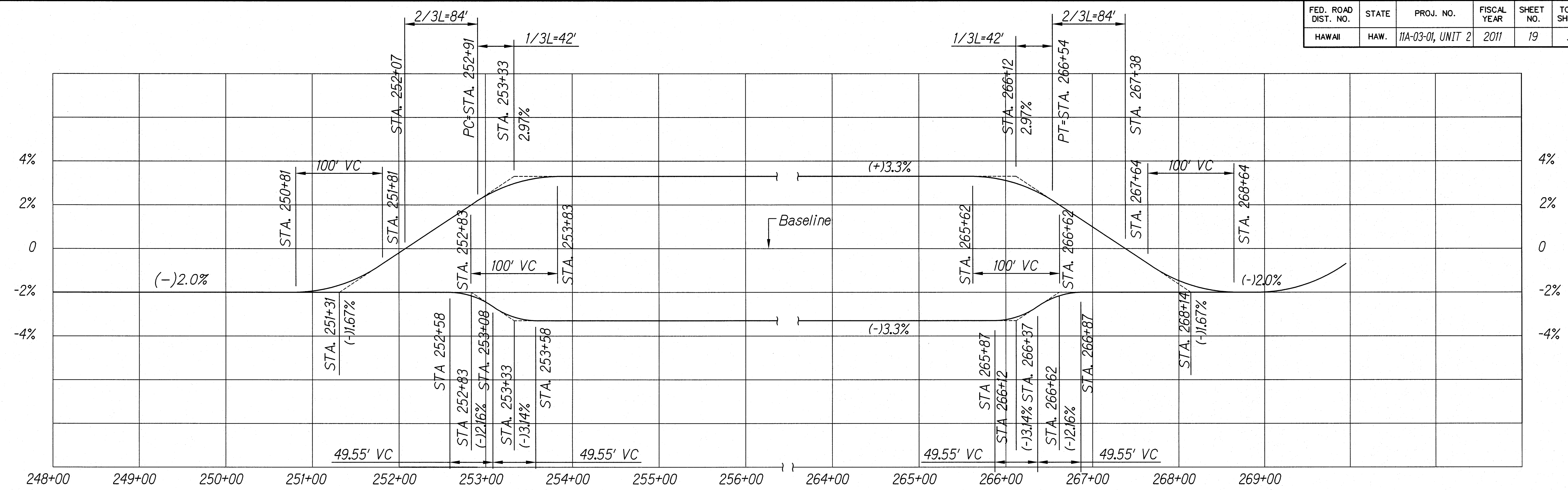
PC STA. 252+91 TO PT STA. 266+54 Scale: Horiz 1"=60' Vert 1"=2%
